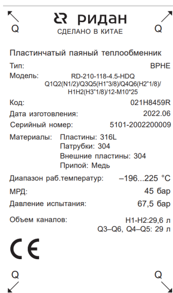
Рис.5 – Пример шильда пластинчатого паяного теплообменника BRHE
