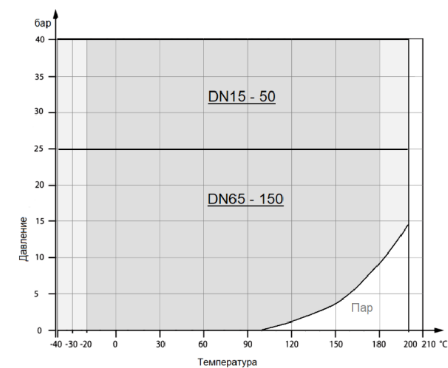
График Температура-Давление
