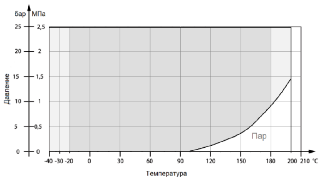
Диаграмма Температура-Давление
