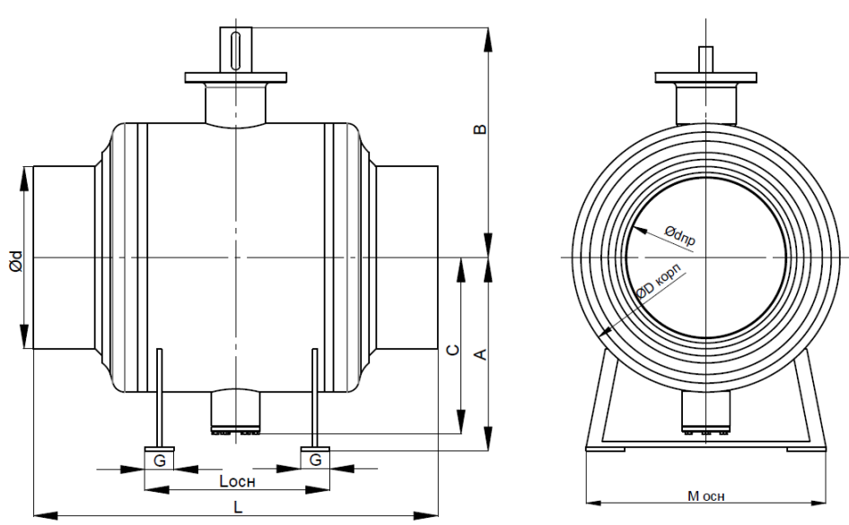
Габаритные и присоединительные размеры кранов шаровых типа RJIP, фланцевые. Дополнительные технические характеристики
