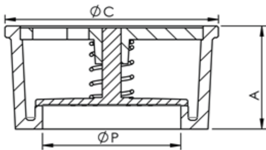
Габаритные и присоединительные размеры обратных затворов. Дополнительные технические характеристики
