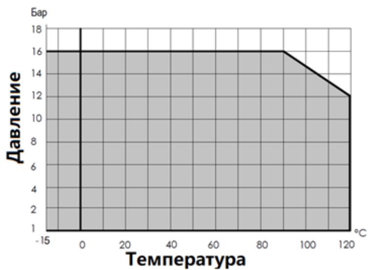
Диаграмма Температура-Давление
