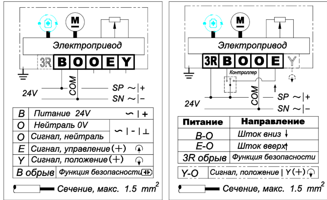
4-проводная схема, Импульсное управление, с аналоговым сигналом обратной связи
