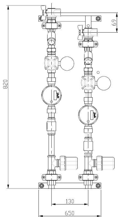
Схема габаритных размеров узла ШКСВ-1Р с правосторонним подключением
