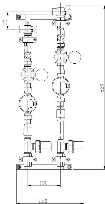
Схема габаритных размеров узла ШКСВ-1Р с левосторонним присоединением
