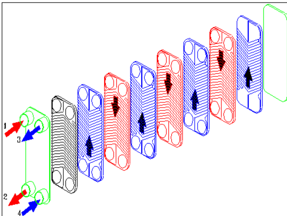
Схема ТО XB
