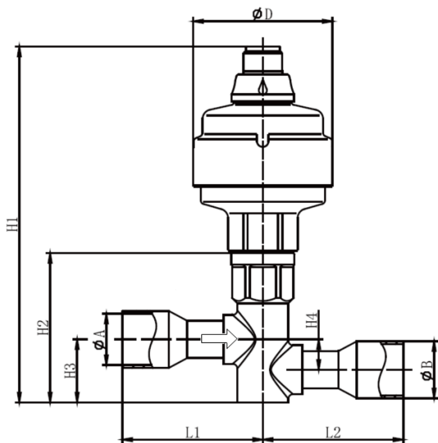
Габариты ETS 50-100.
