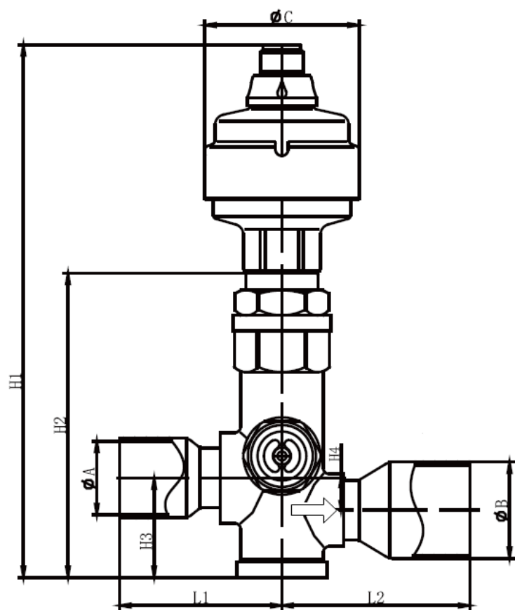
Габариты ETS 250-400.
