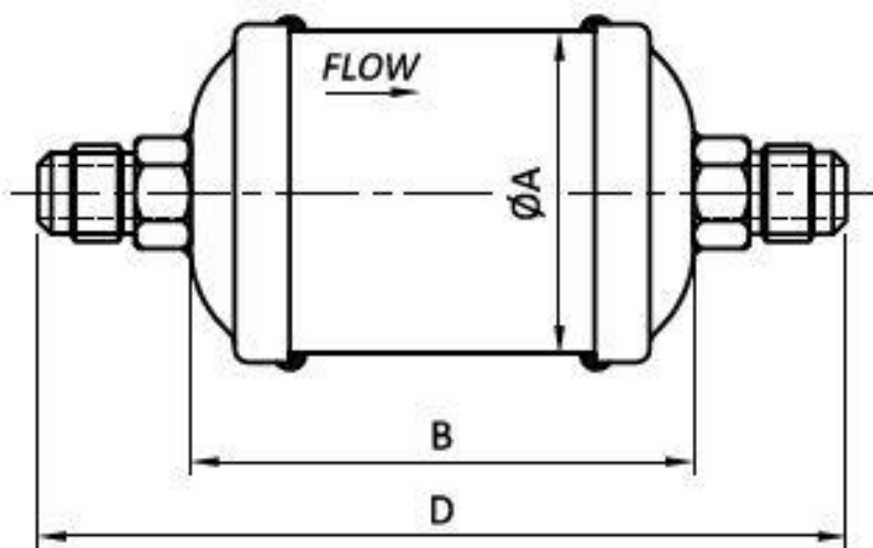
Типоразмер DGL 05-41
