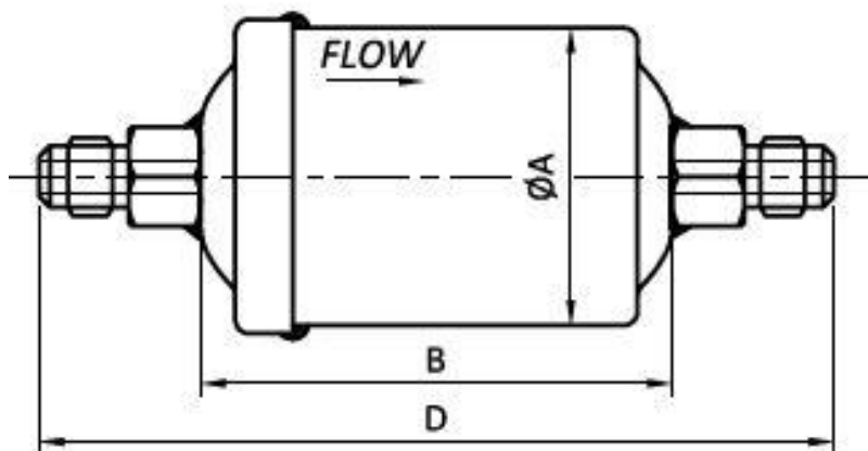
Типоразмер DGL 05-41
