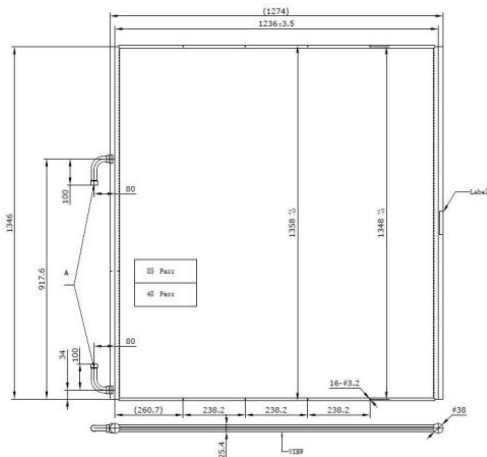
Габаритные размеры и изображение теплообменника микроканального модификации RC-1900.
