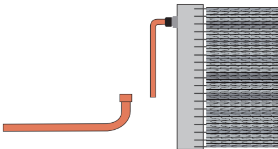
Рис. 2 – Корректное подключение к патрубкам
