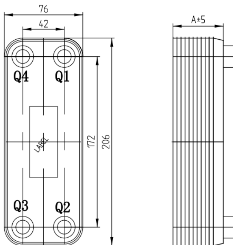
Рис.6 - Габаритные размеры и изображение теплообменника пластинчатого модификации BPHE_RD-014
