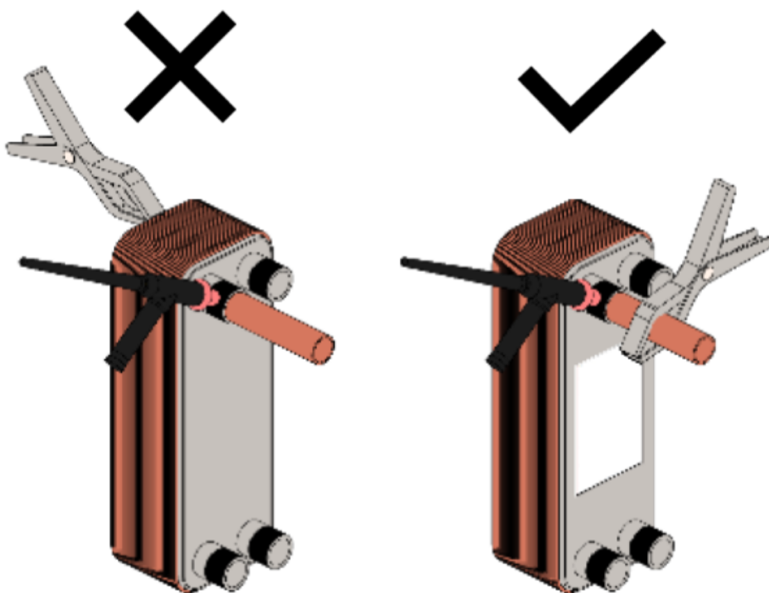
Рис.10 - Подключение клеммы заземления во время электросварки
