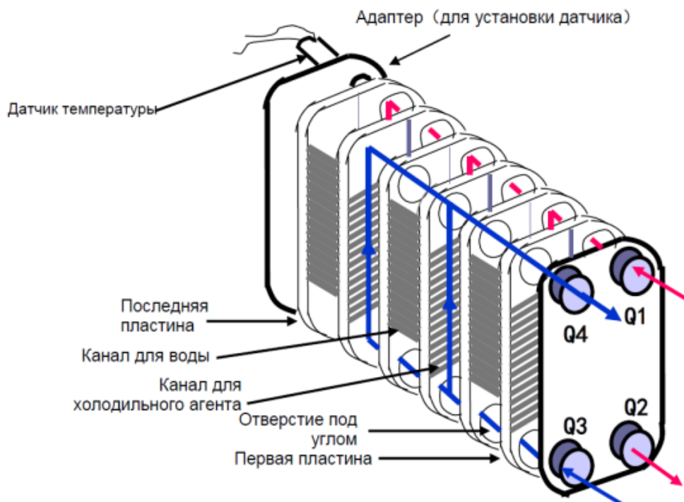
Рис.3 - Схема теплообменника пластинчатого типа BPHE.
