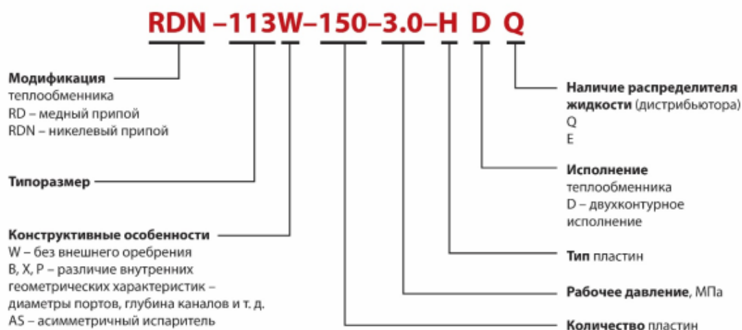
Рис.4 - Пример условного обозначения теплообменников пластинчатых типа BPHE
