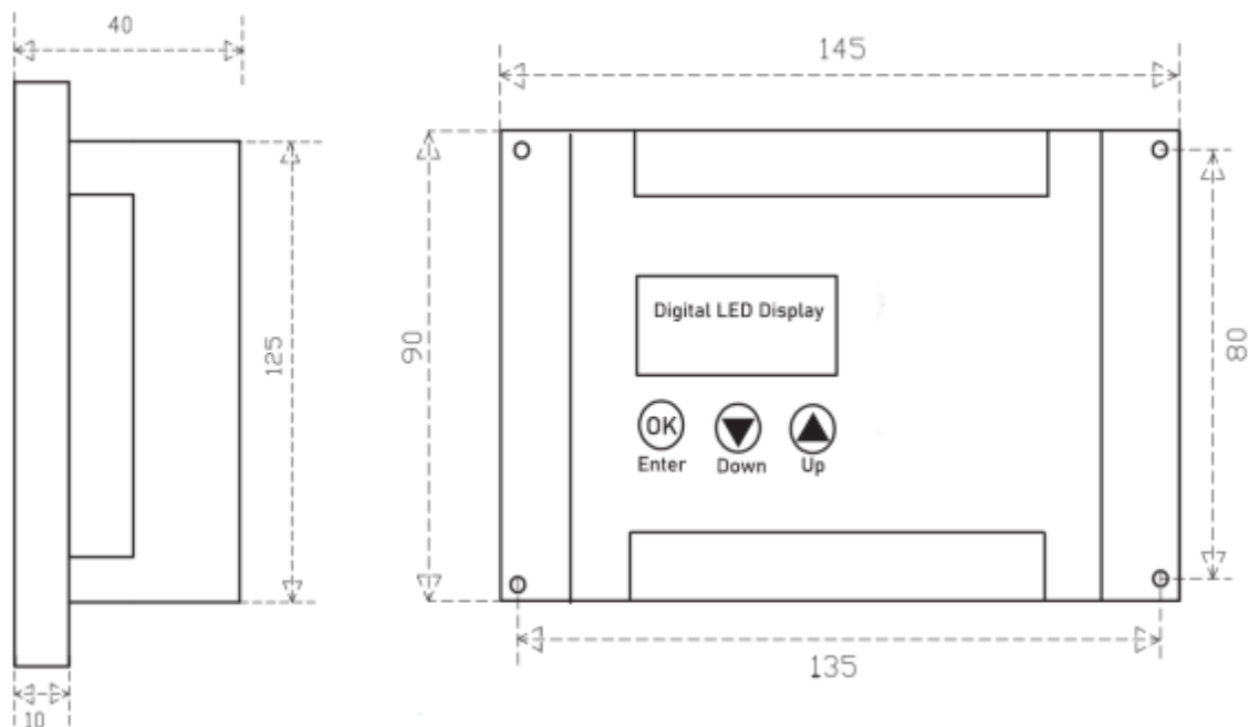
Габаритные размеры контроллеров типа Р-КИ
