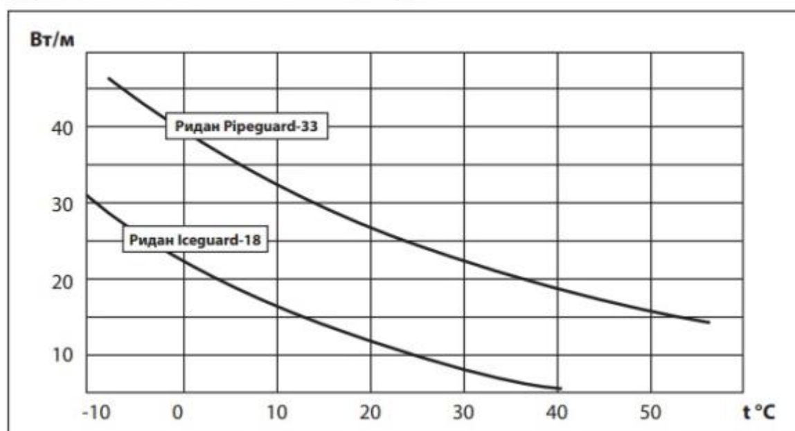
Теплоотдача саморегулирующихся кабелей на металлической трубе в зависимости от температуры
