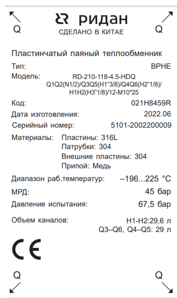
Рис.5 – Пример шильда пластинчатого паяного теплообменника БРНЕ
