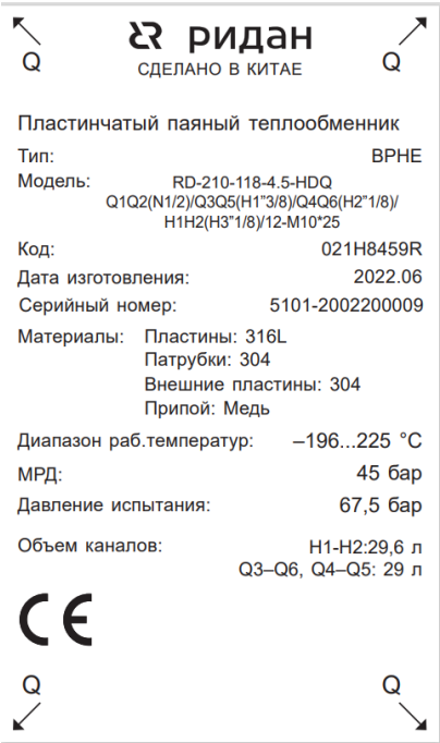
Рис.5 – Пример шильда пластинчатого паяного теплообменника VRHE
