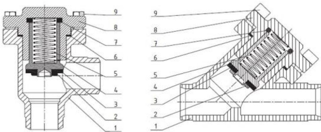
Рис. 1 – Конструкция клапана
