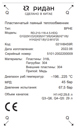
Рис.5 – Пример шильда пластиначатого паяного теплообменника ВРНЕ
