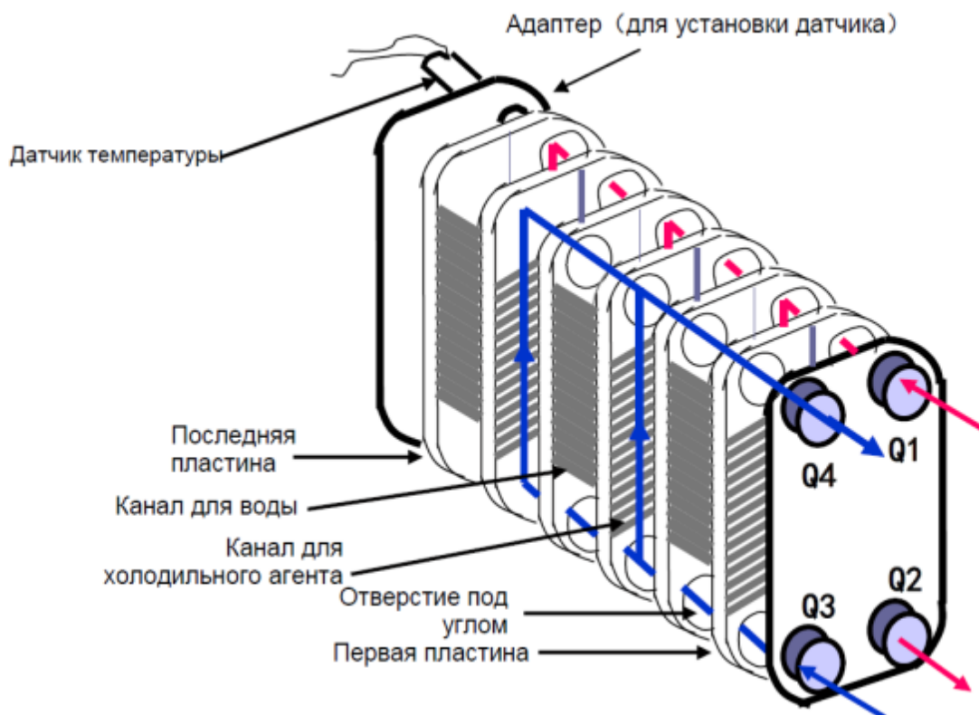
Рис.3 - Схема теплообменника пластинчатого типа BPHE.
