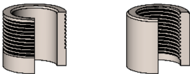
Рис.8 - Резьбовые соединения
