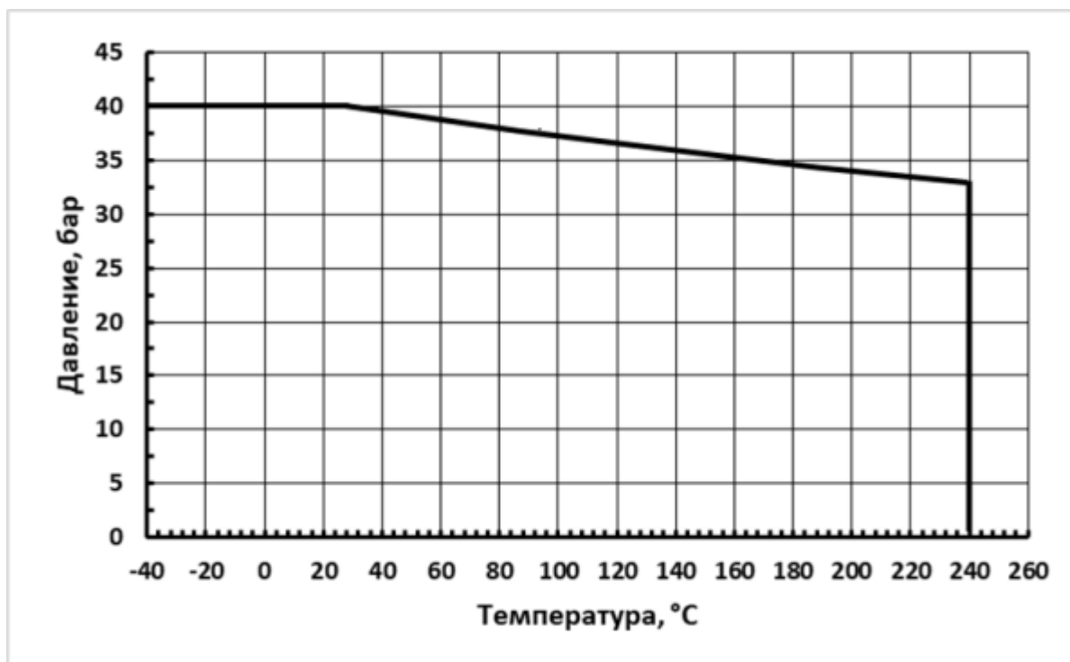
Диаграмма Температура-Давление
