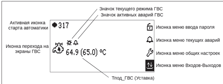
Рис. 6. Главный экран ECL3R 317 FC.
