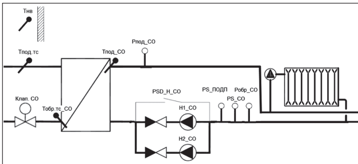
Рис. 2. Схема и параметры СО
