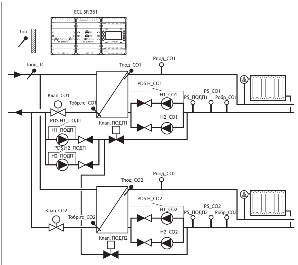
Рис. 1. Схема приложения регулятора ECL-3R 361
