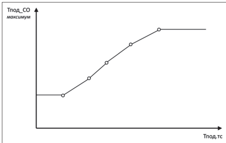
Рис. 8. Ограничение T_{под\_СО} от T_{под.тс}
