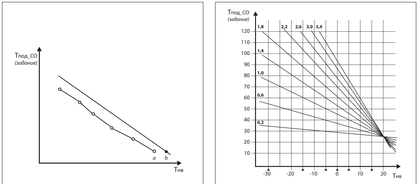
Рис. 4. Два варианта задания отопительного графика: график по точкам (а) и через угол наклона (b)
