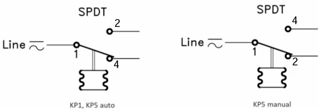
Однополюсная двухпозиционная контактная группа SPDT
