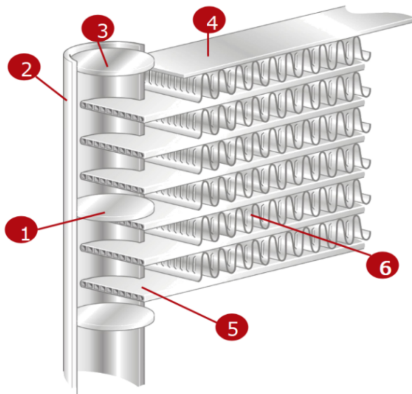
Устройство теплообменников микроканальных типа МСНЕ.
