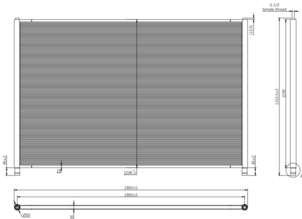
Габаритные размеры и изображение теплообменника микроканального модификации RF-1950.
