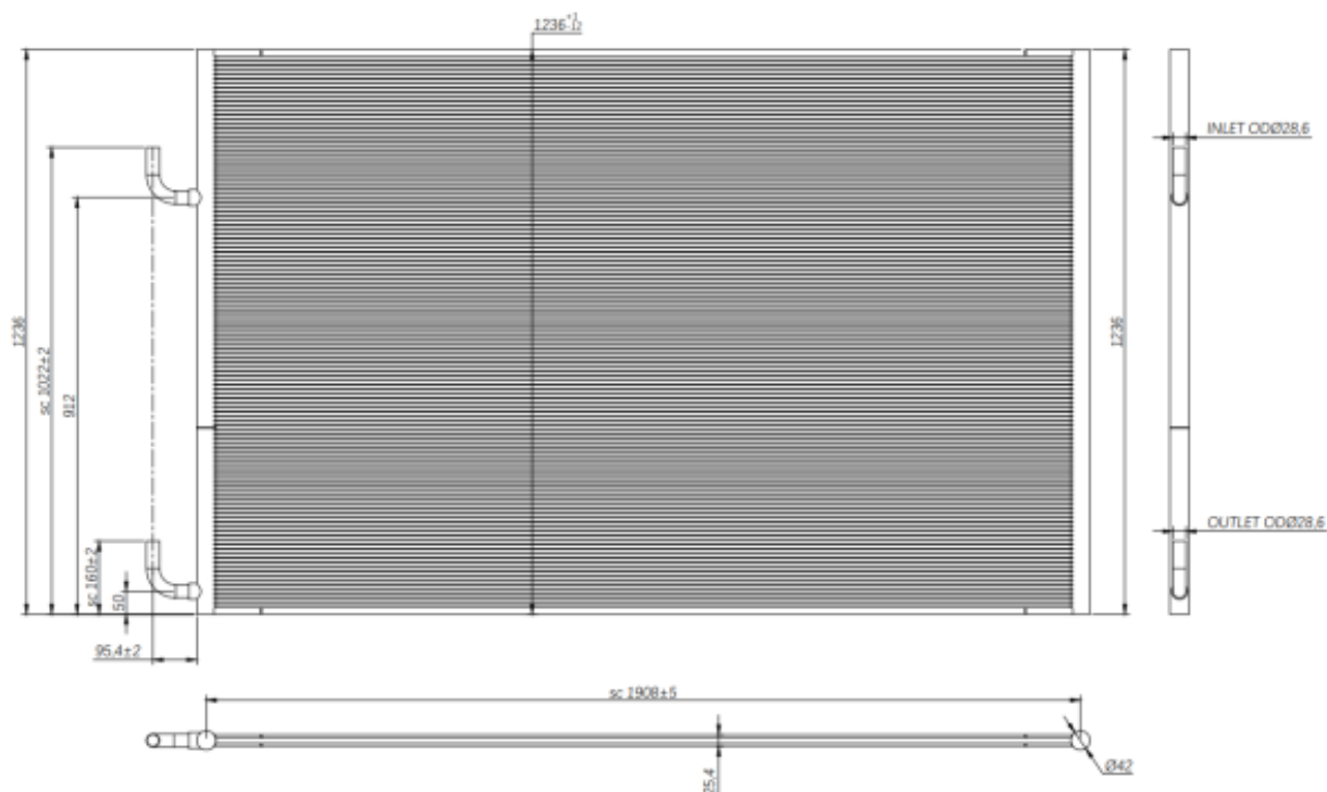
Габаритные размеры и изображение теплообменника микроканального модификации RF-1950.
