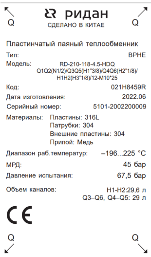
Рис.5 – Пример шильда пластинчатого паяного теплообменника VRHE
