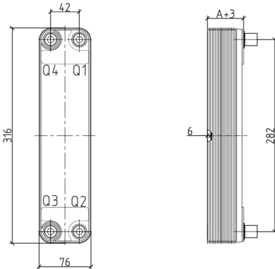
Рис.6 - Габаритные размеры и изображение теплообменника пластинчатого модификации VRHE_RD-020
