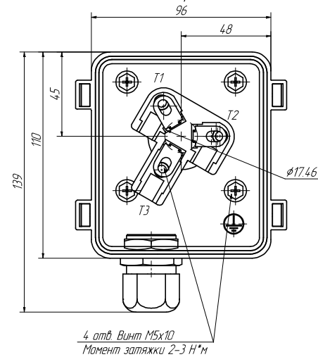
Клеммная коробка (1:1)
