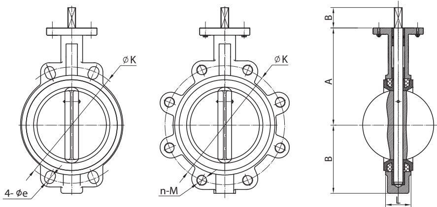
Ридан 3ДМ с рукояткой
