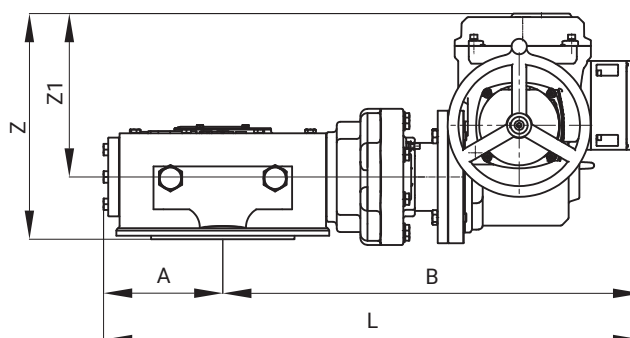
Электроприводы АМВ-М (без блока местного управления)
