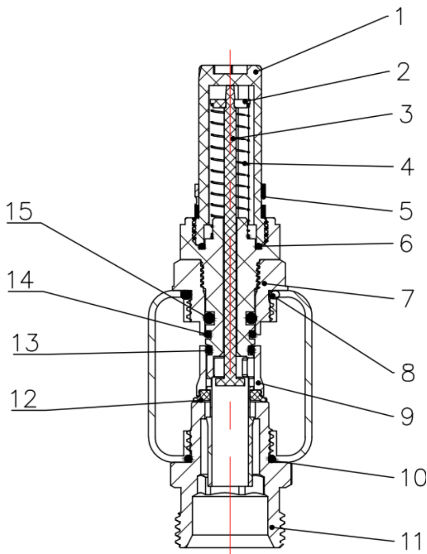
Рис. 1. Устройство подающей гребенки с ротаметрами
