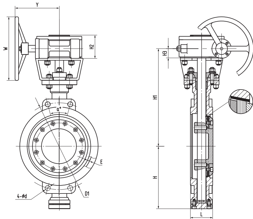
Межфланцевый дисковый затвор с редуктором
