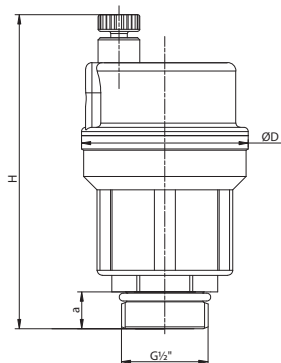
Автоматический воздухоотводчик Airvent-R без обратного клапана
