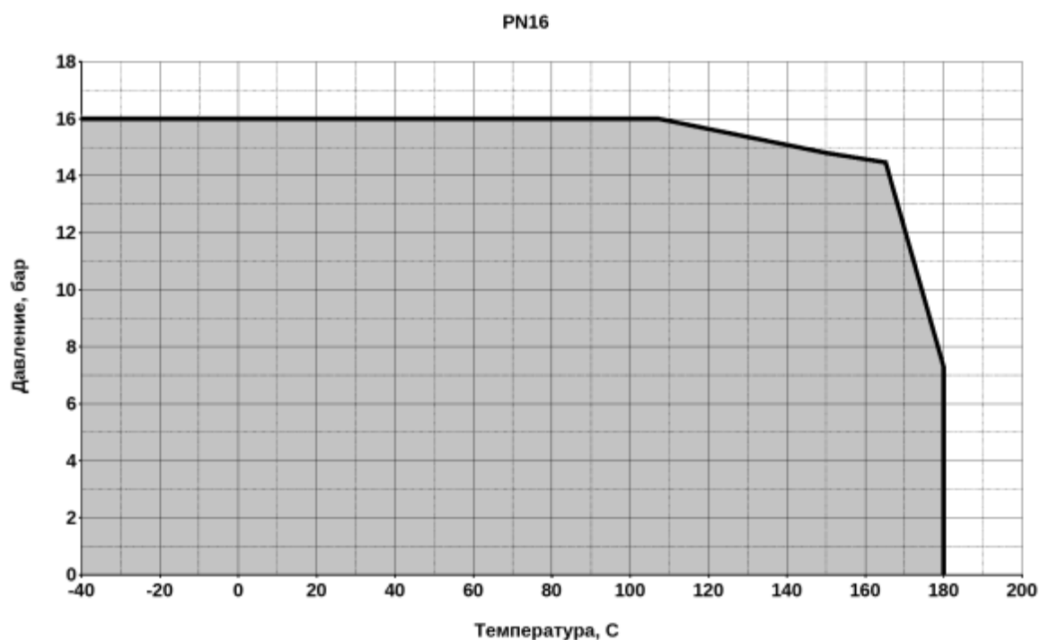
Диаграмма Температура-Давление
