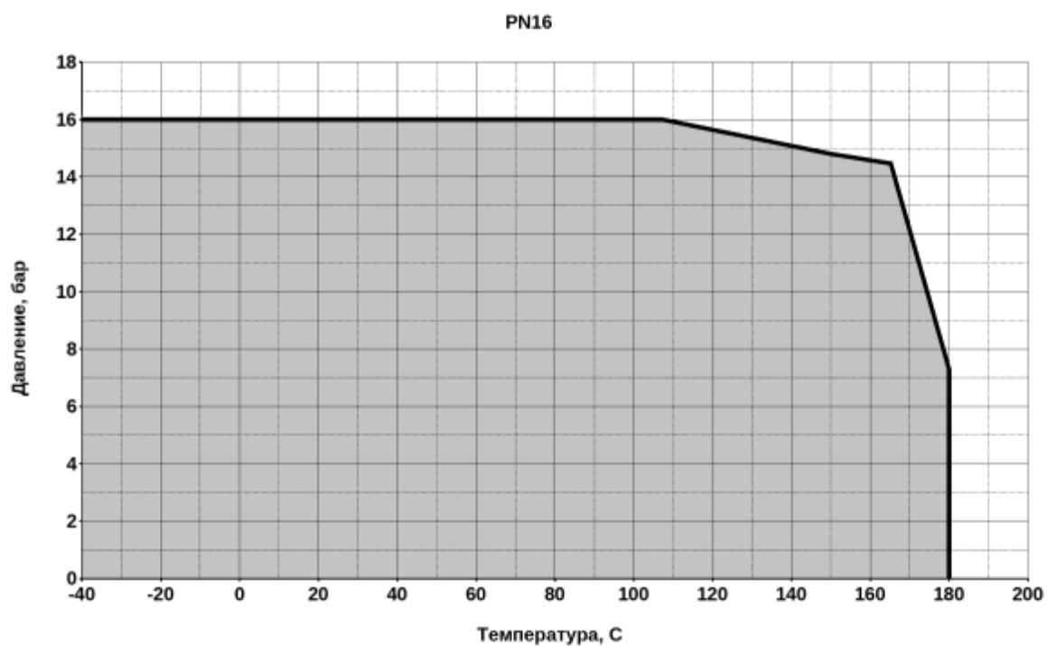
Диаграмма Температура-Давление
