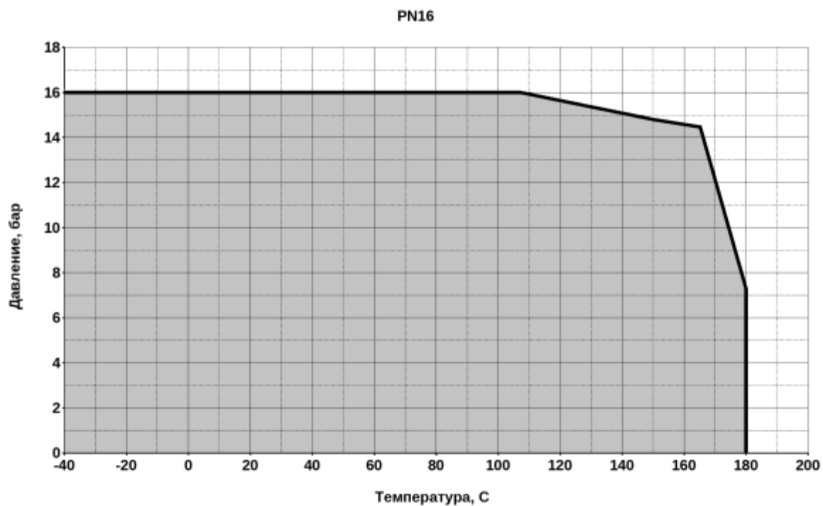
График Температура-Давление
